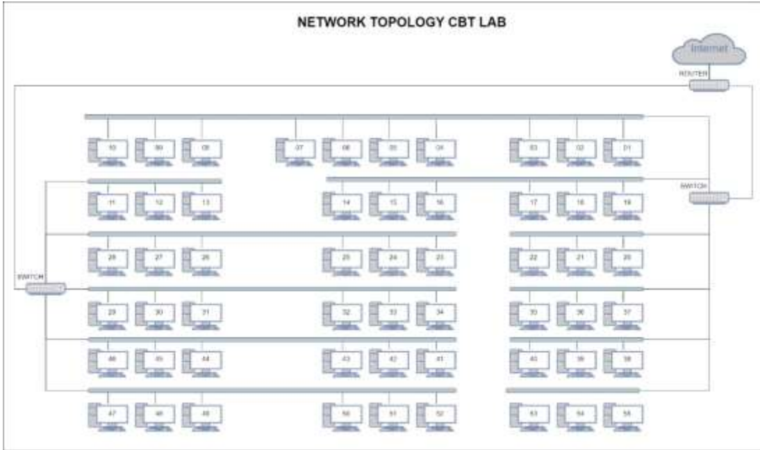
Gambar topologi LAN ruangan cbt
